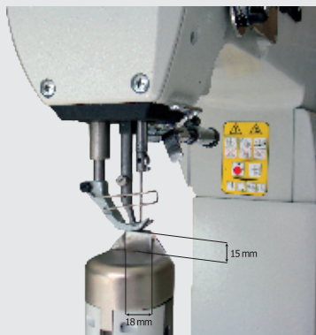
Particolare degli organi di cucitura Sewing parts detail
